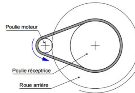
Schéma du système de propulsion
